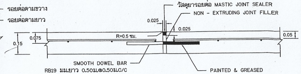
ขยายรอยต่อ EXPANSION JOINT
