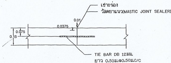
ขยายรอยต่อ LONGITUDINAL JOINT
