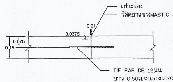
ขยายรอยต่อ LONGITUDINAL JOINT
