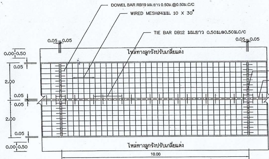
รูปแบบแสดงการเสริมเหล็กและรอยต่อ
