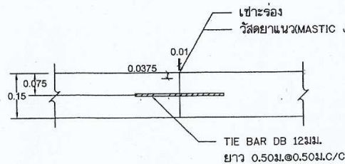
ขยายรอยต่อ LONGITUDINAL JOINT
